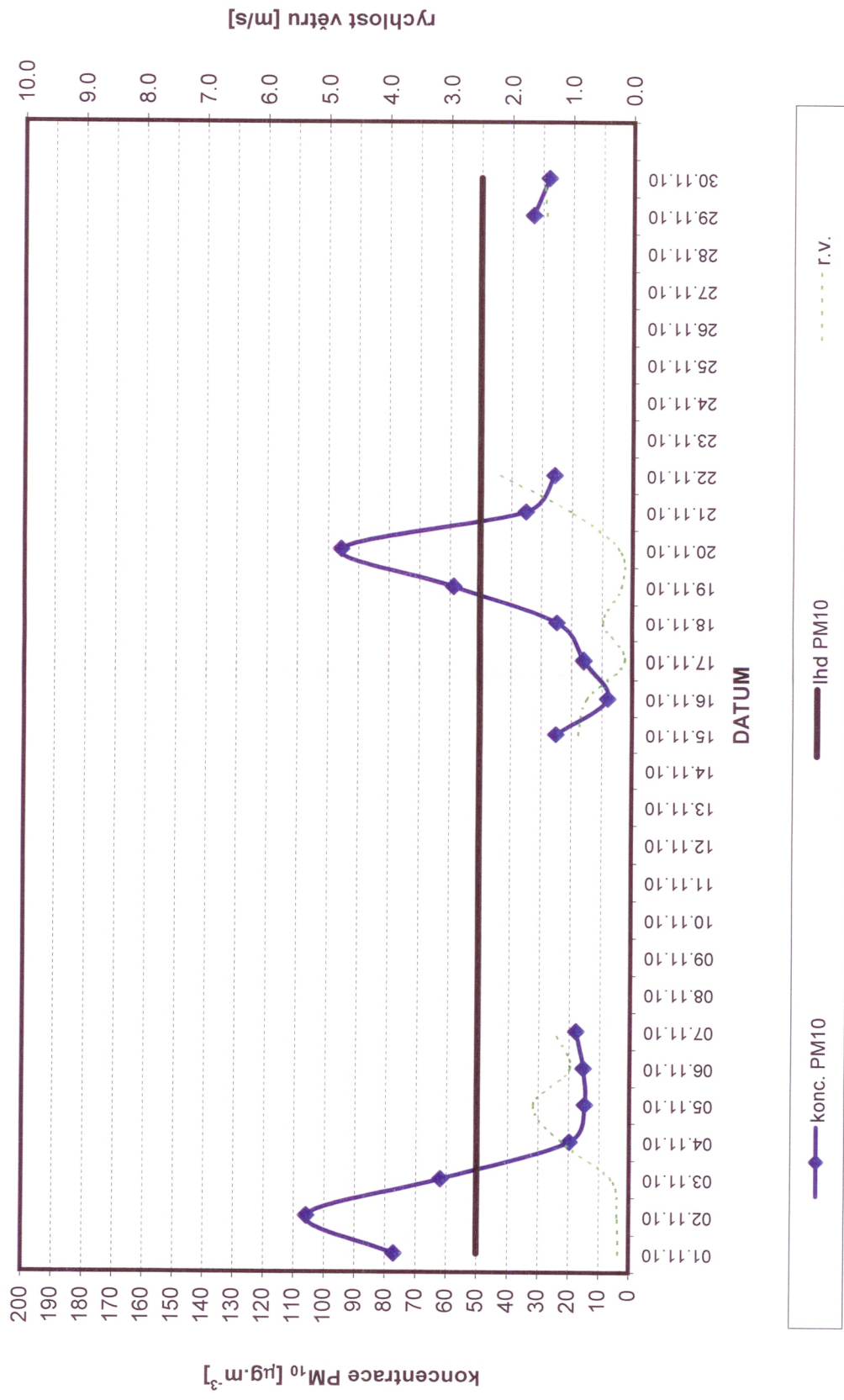
Průběh průměrných denních koncentrací suspendovaných částic PM_{10} ve volném ovzduší a hodnot rychlosti větru (r.v.)
